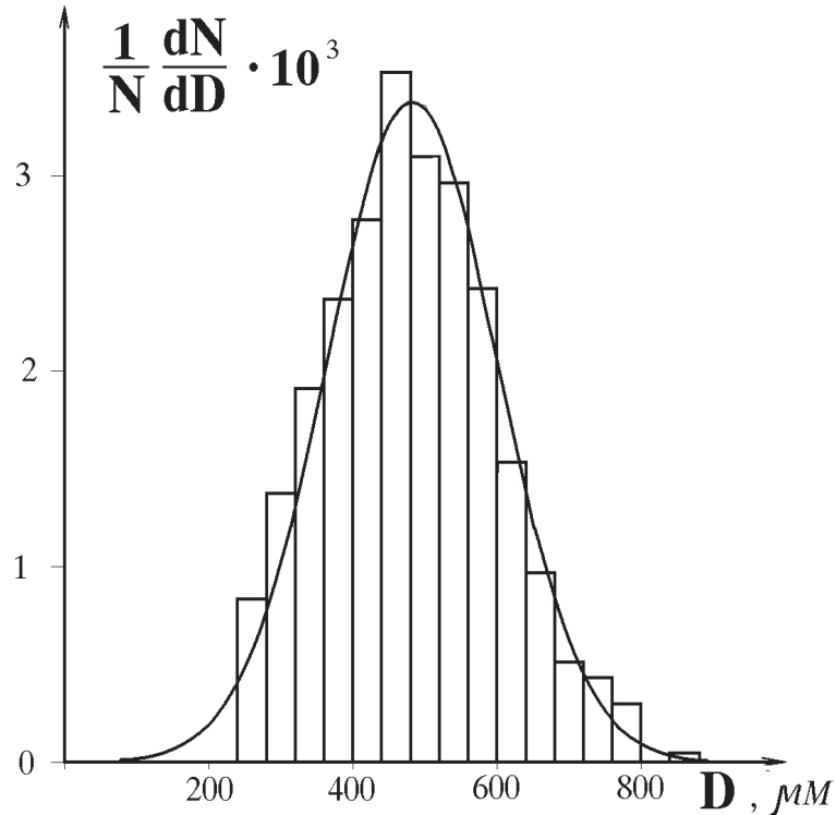
Рис. 2. Гистограмма распределения глубины испарения графитовой пластины в эксперименте на ГОЛ-3
